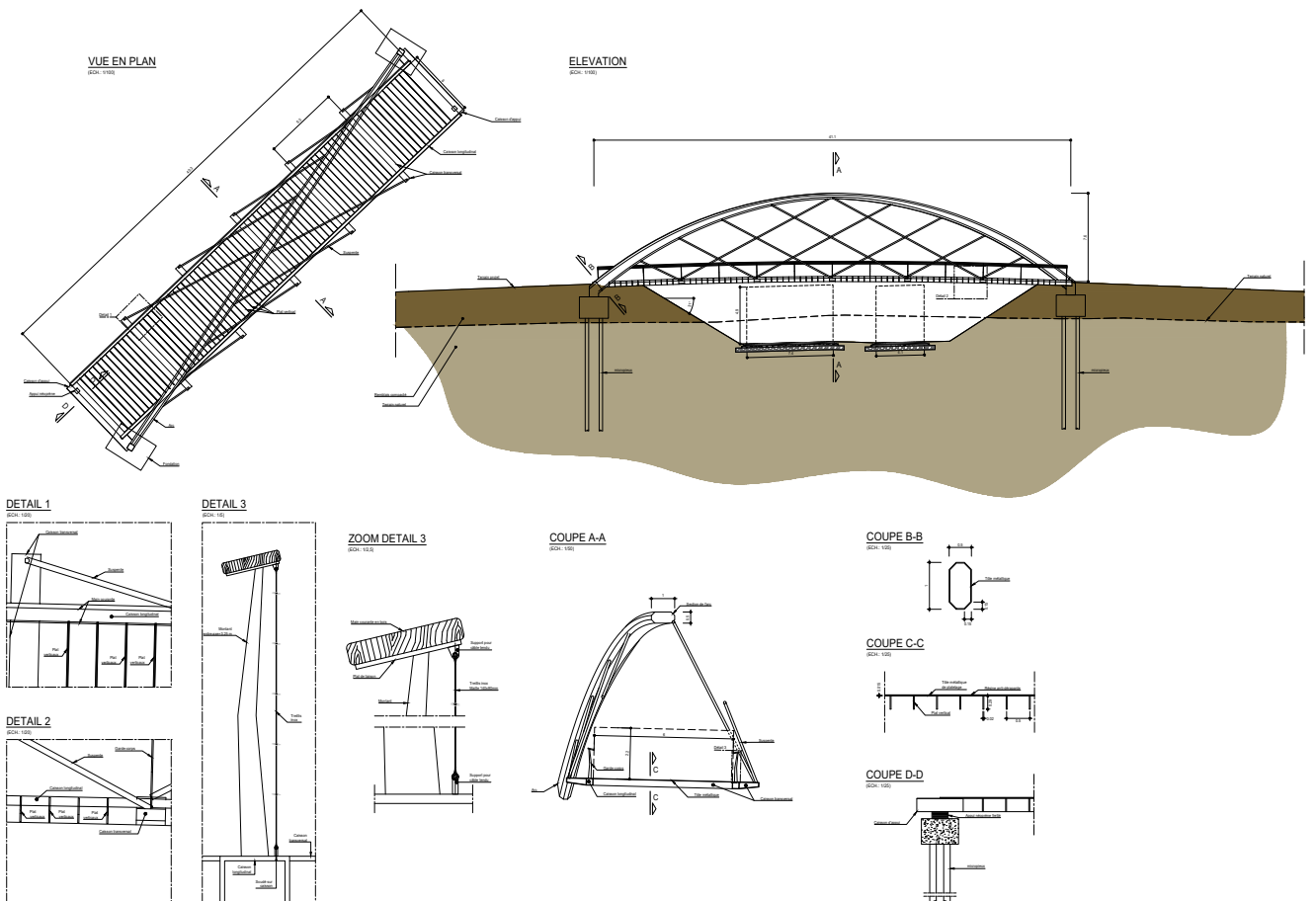
Détail et coupe type de la passerelle cyclo-piétonne (par le Bureau d'études Greisch)
